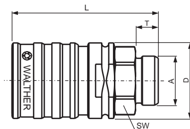
Муфта с клапаном / Self sealing coupling
