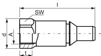
ниппель с клапаном self sealing adaptor
