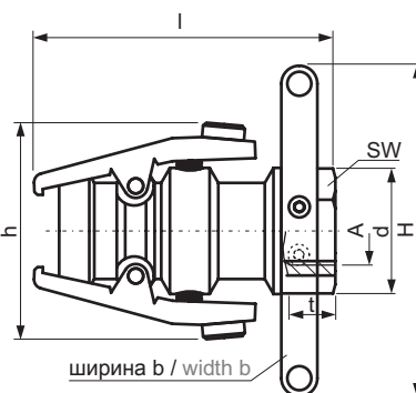
муфта с клапаном self sealing coupling
