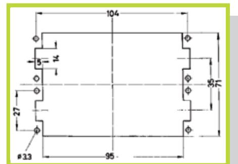
Dima di foratura per inserti senza custodia Panel cut out
