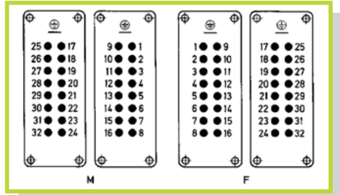
Disposizione dei contatti (vista lato cavi) Contact arrangement (view from termination side)
