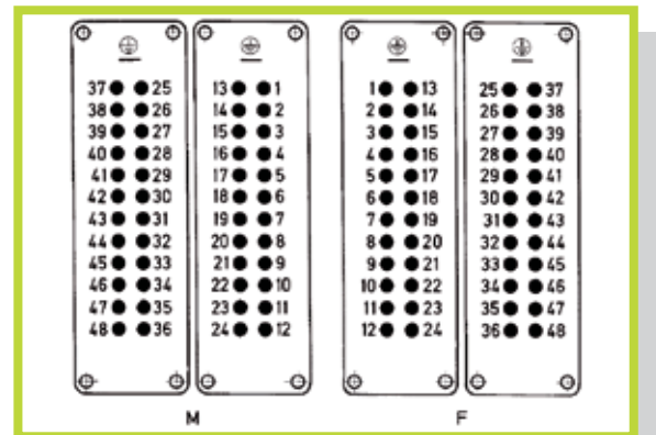
Disposizione dei contatti (vista lato cavi) Contact arrangement (with termination side)
